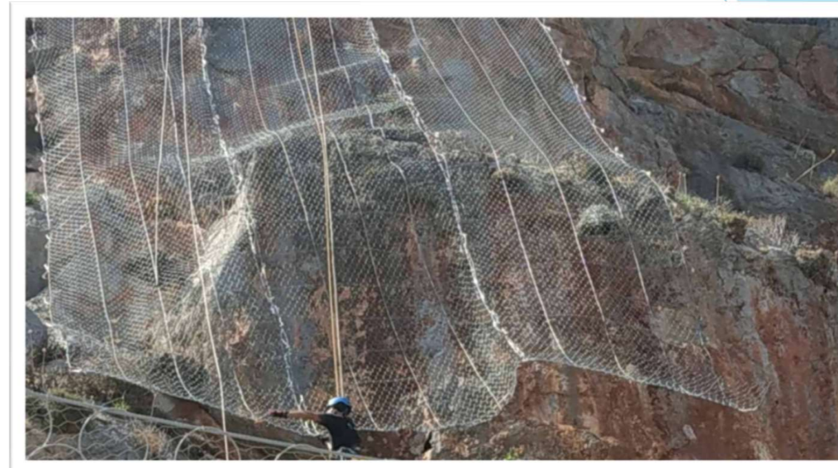
06/2022 | Εγκατάσταση πλέγματος επένδυσης πρανών
