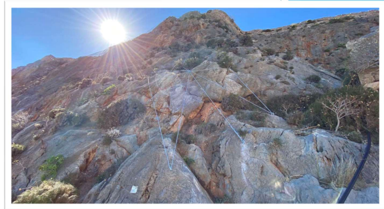
05/2022 | Περιδέσεις βραχωδών τεμαχών
