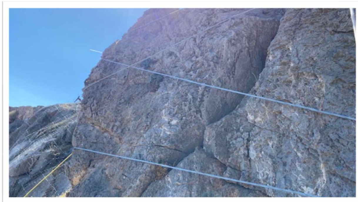
05/2022 | Περιδέσεις βραχωδών τεμαχών
