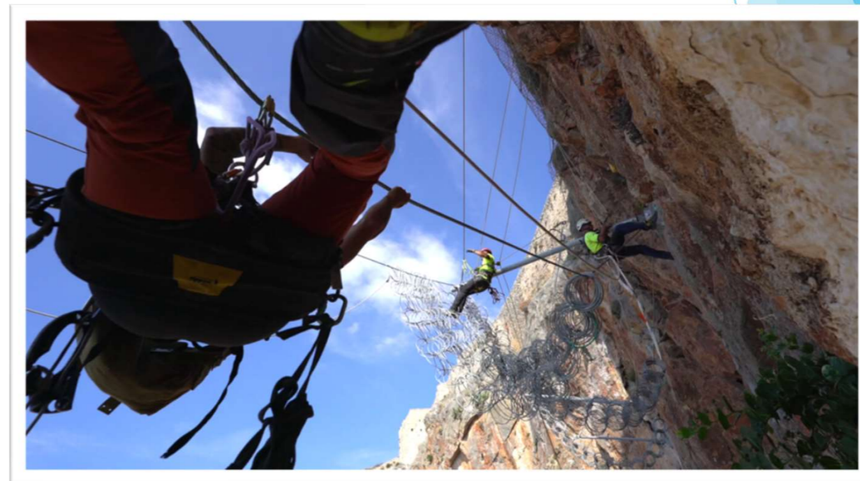
06/2023 | Ανάρτηση - Τάνυση πλέγματος φραχτών ανάσχεσης
