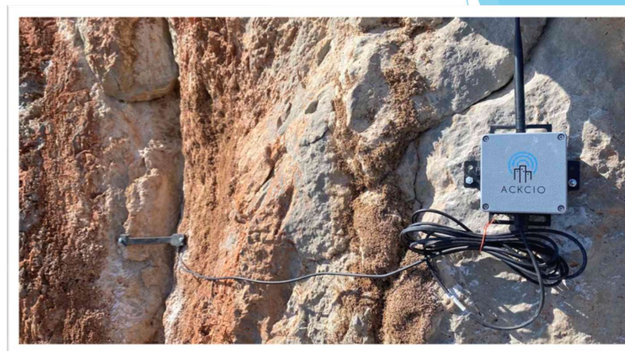
06/2023 | Εγκατάσταση ασύρματου ηλεκτρικού ρωγμόμετρου
