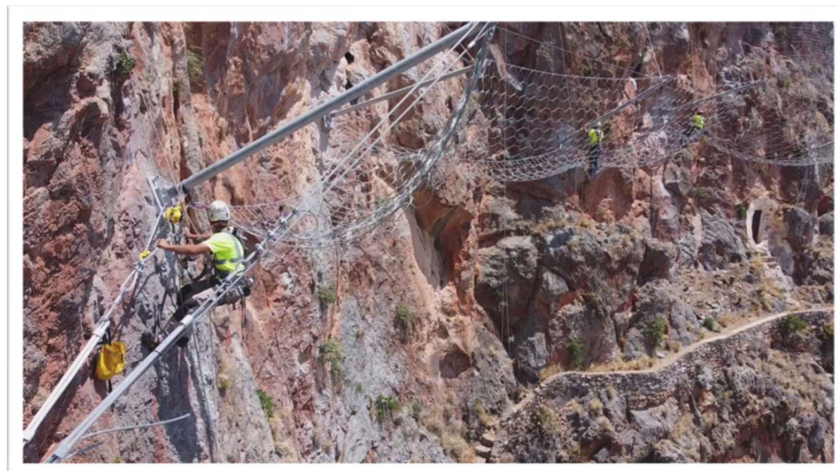
06/2023 | Ανάρτηση - Τάνυση πλέγματος φραχτών ανάσχεσης
