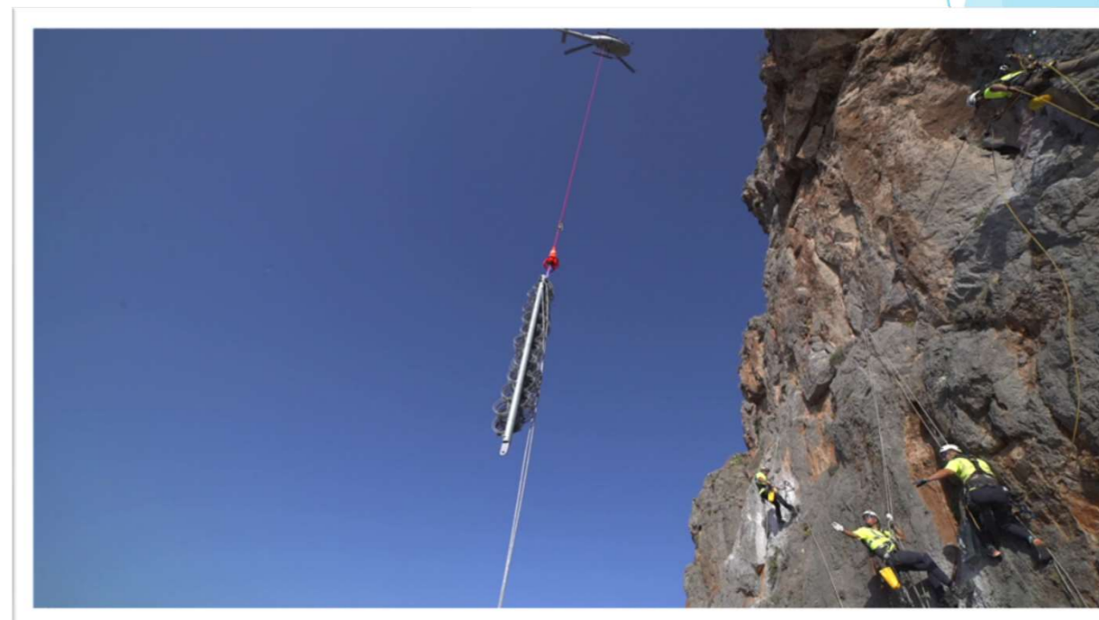
05/2022 | Μεταφορά φραχτών ανάσχεσης με χρήση ελικοπτέρου
