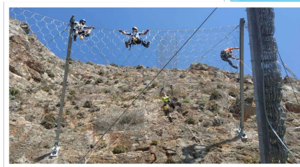
06/2022 | Ανάρτηση - Τάνυση πλέγματος φραχτών ανάσχεσης
