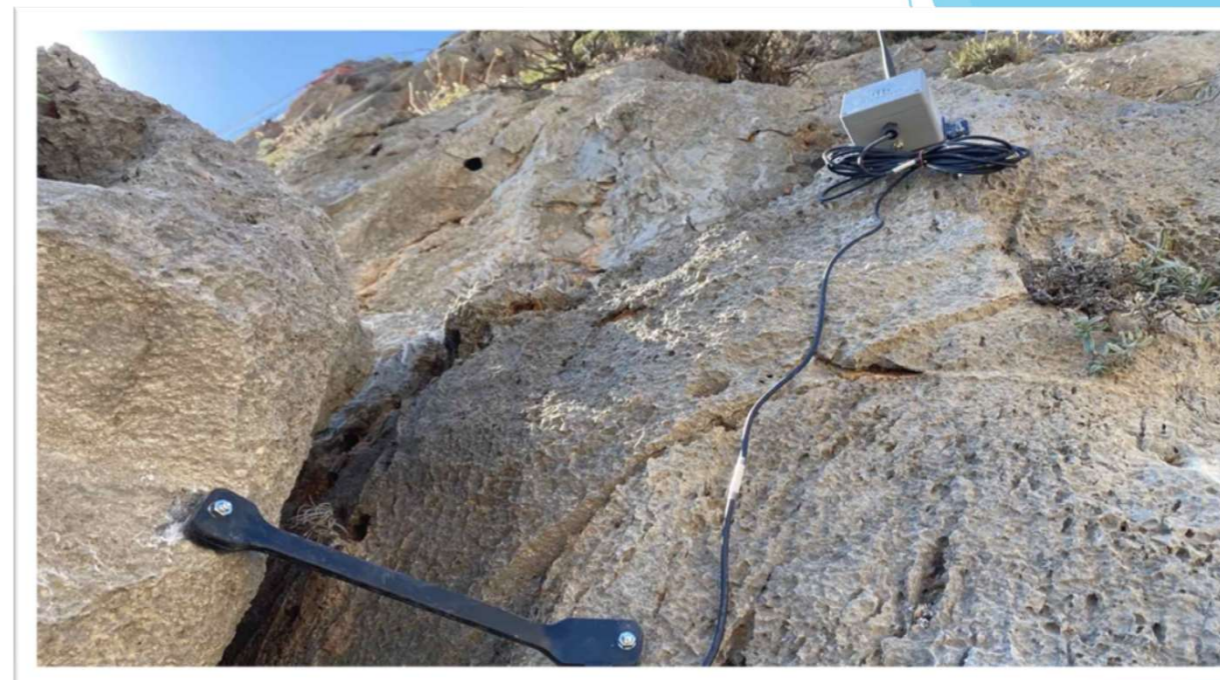
10/2022 | Εγκατάσταση εξοπλισμού ασύρματης τηλεπαρακολούθησης
