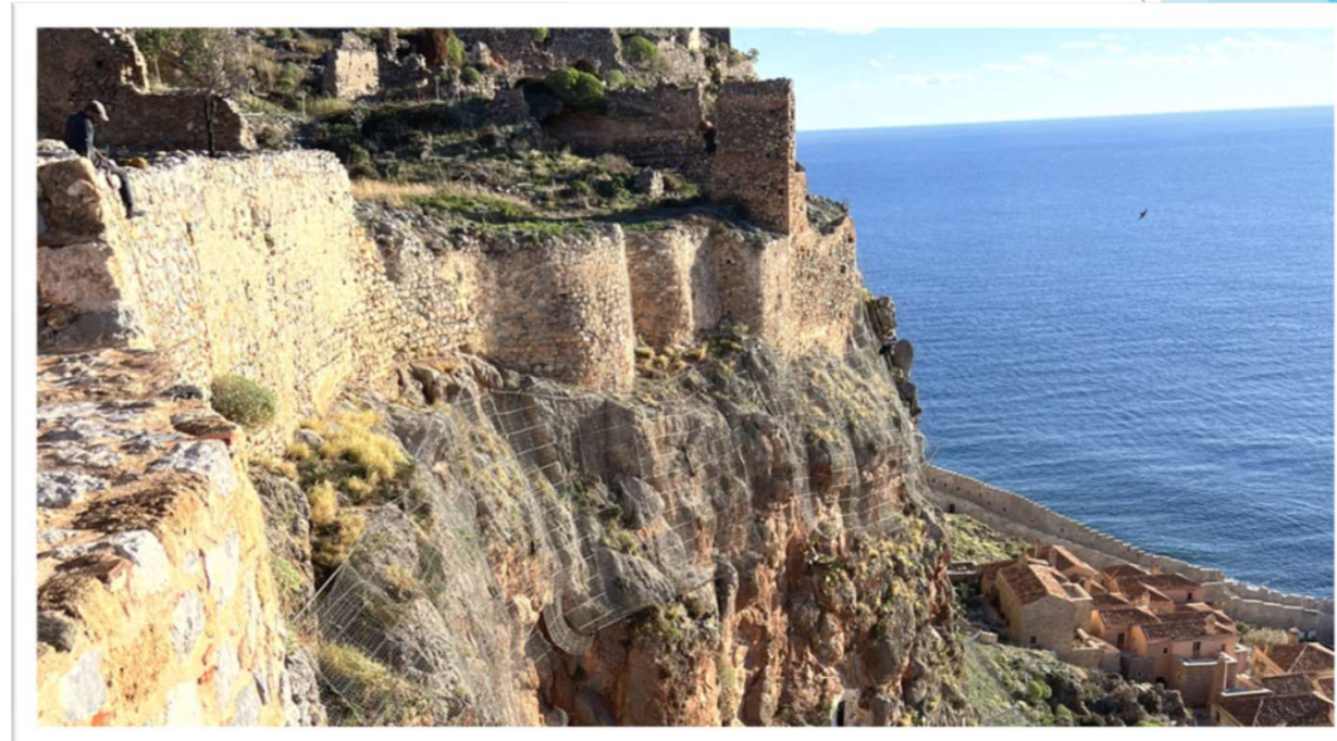
06/2023 | Ολοκλήρωση εργασιών σταθεροποίησης βραχωδών πρανών
