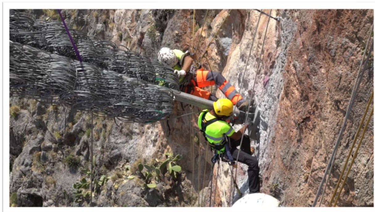
05/2022 | Εγκατάσταση φραχτών ανάσχεσης με χρήση ελικοπτέρου
