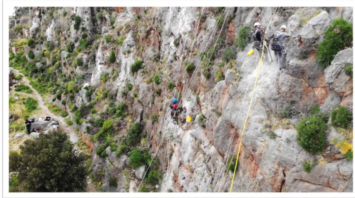
03/2022 | Διατρήσεις βράχων - εγκατάσταση αγκυριών
