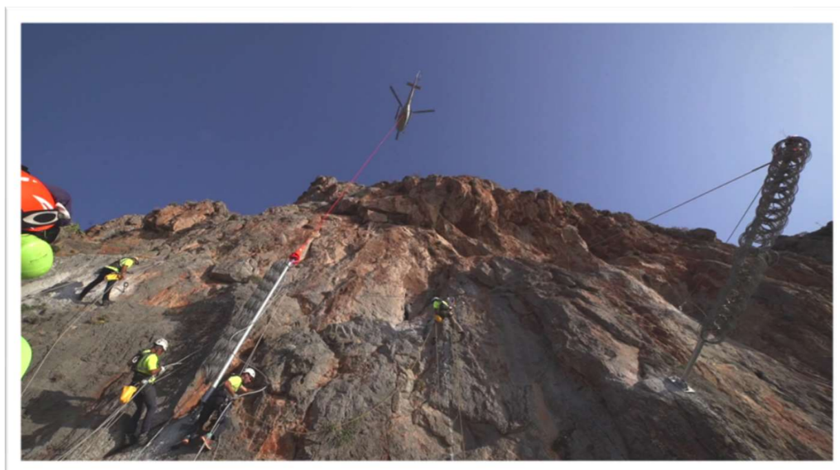
05/2023 | Εγκατάσταση φραχτών ανάσχεσης με χρήση ελικοπτέρου
