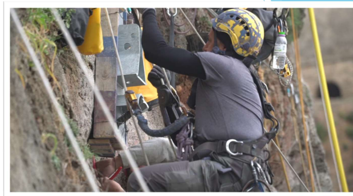
04/2022 | Κατασκευή βάσεων φραχτών ανάσχεσης βραχοπτώσεων
